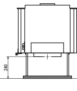
背面図
