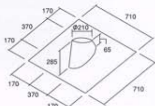
フラッシング30°以上 (アルミ)
