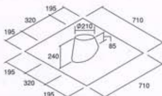
フラッシング30°以下 (アルミ)
